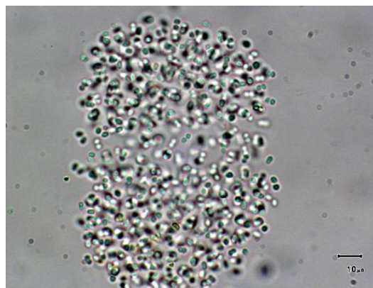
Aphanocapsa
