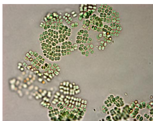
Merismopedia
