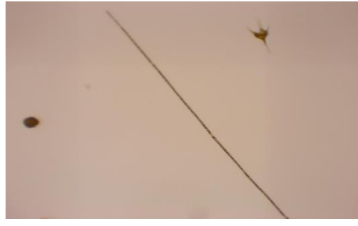
Dolichospermum/Anabaena
