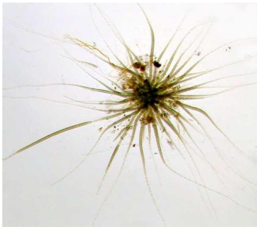
Gloeotrichia
