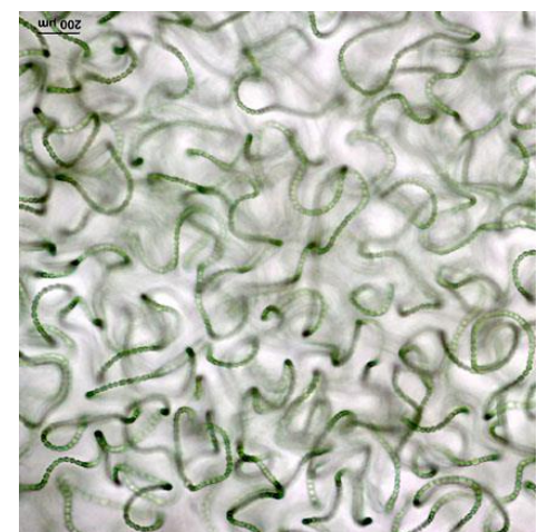
Nostoc
