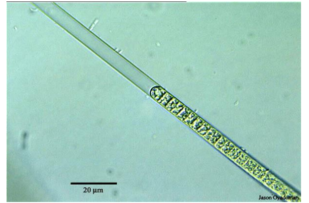
Lyngbya
